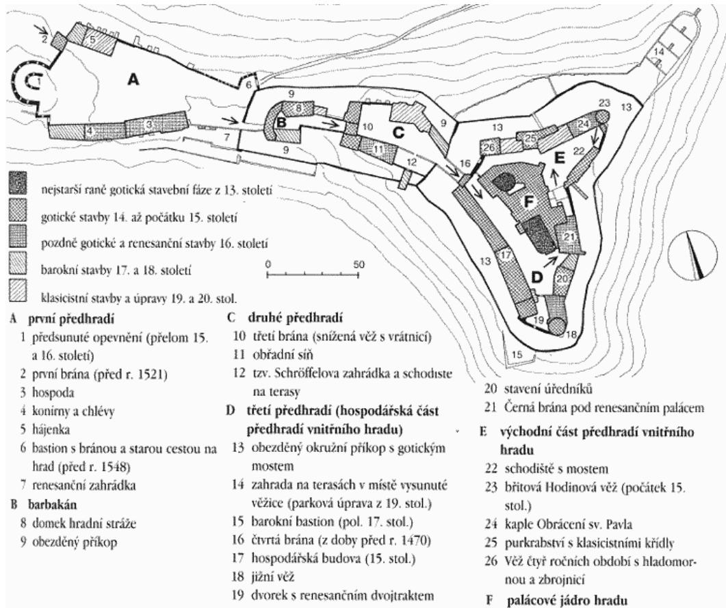
Obr. 3: Půdorys hradu
